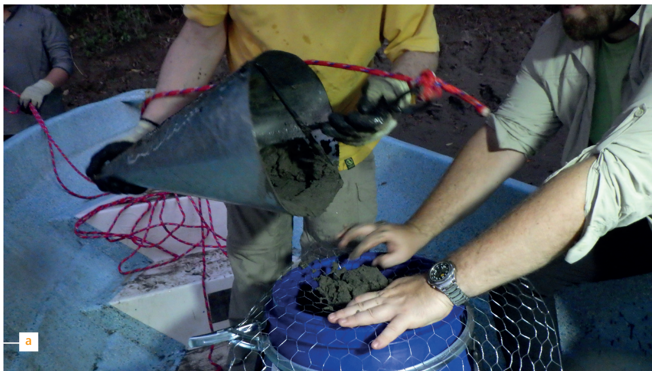
Figure 4.2 : Prélèvements manuels des sédiments de l'Usumacinta : (a) avec cône, (b) avec pelle, (c) avec seau. © I. Djeran-Maigre, avril 2018.
