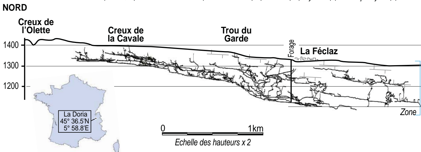
Figure 2 : Vue en coupe du réseau karstique souterrain du plateau de la Féclaz (d'après carte spéléologique au 1/10 000 Spéléo Club de Savoie). Cross-Sectional view of the underground karstic system of the Feclaz (according to Speleo-Club de Savoie speleological map at 1/10,000)
